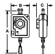
轻型 (BL系列)
