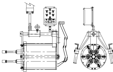
水平前支撑 (轮母应用)
