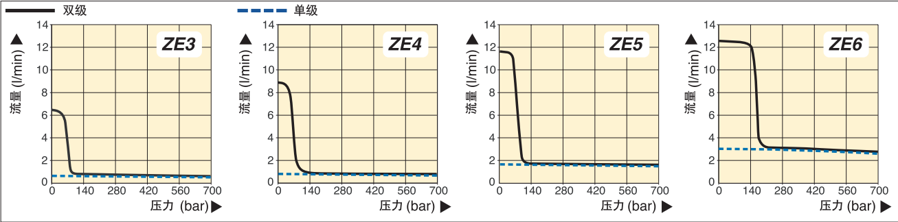
▼ZE系列泵性能表
