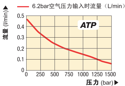
流量图
